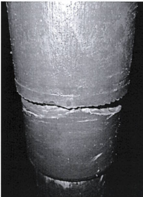
1.2. Нижняя часть разрушившейся муфты НКТ скважины № 4-3 ВУ ОНГКМ в зацеплении с труболовкой
