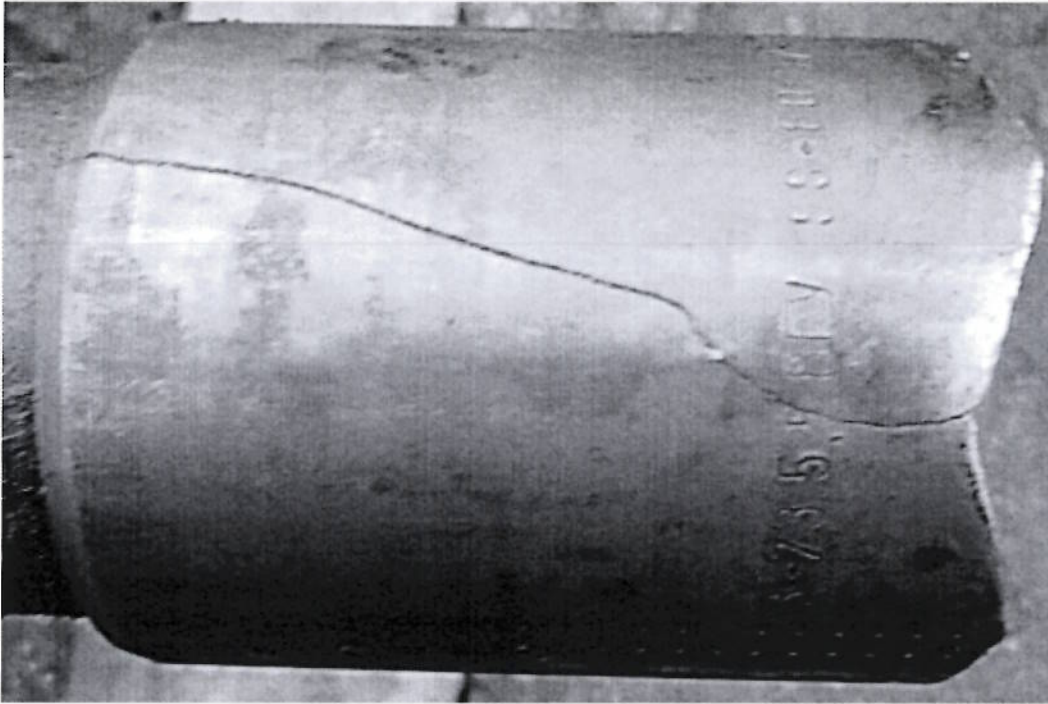
1.1. Верхняя часть разрушившейся муфты НКТ скважины № 4-3 ВУ ОНГКМ с трещиной
