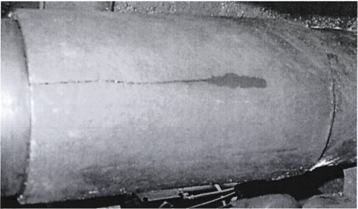
1.3. Муфта НКТ скважины № 1294 ВУ ОНГКМ с трещиной
